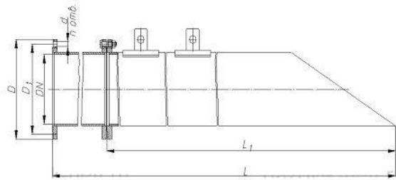
Общий вид трубы подъемной ТП
