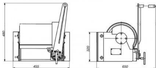
Общий вид лебедки ручной ЛР-1000.
