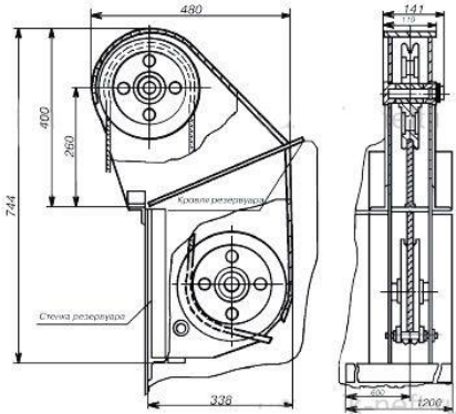
Общий вид блока роликового БР
